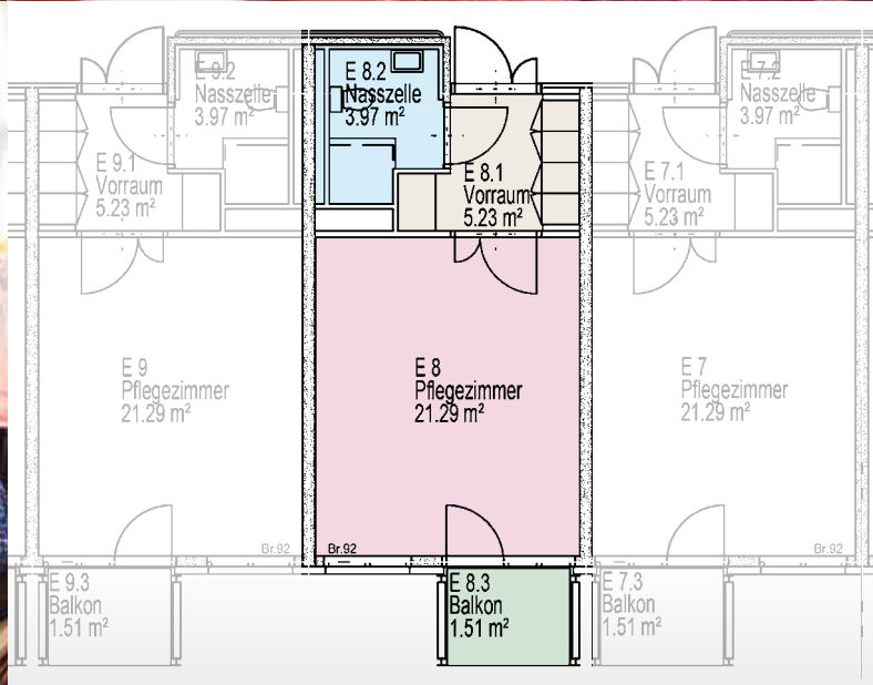
Beispiel Grundriss eines Bewohnerzimmers
